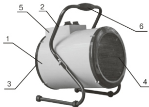
Рис. 1 тепловая пушка
