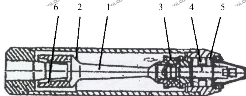
Рис. 3. Вибронаконечник ИВ – 116.01.000 СБ вибратора ВИ – 1-16. 1 – бегунок; 2 – корпус; 3 – муфта упругая; 5 – шпиндель; 5 – подшипник; 6 – сердечник
