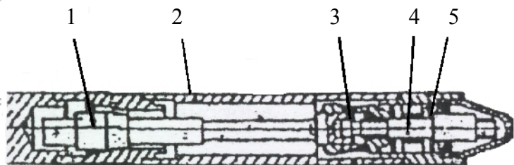
Рис. 4. Вибронаконечник ИВ-113.01.000 СБ, ИВ-117.01.000 СБ вибратора ВИ-1-17, ВИ-1-13, ВИ-75 1 – бегунок; 2 – корпус; 3 – муфта упругая; 4 – шпindelь; 5 – подшипник
