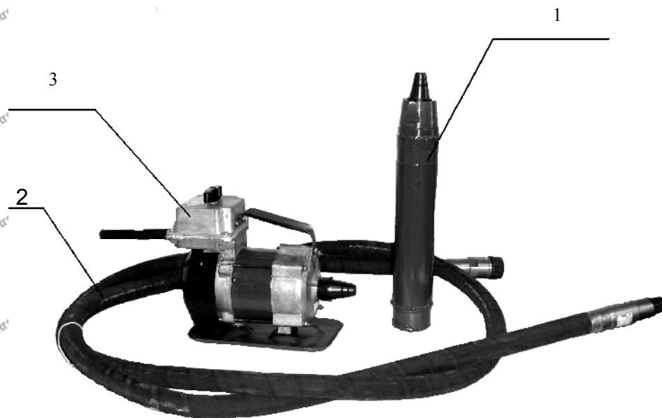
Рис.1. Вибраторы ручные электрические глубинные с гибким валом ВИ-1-16, ВИ-1-17, ВИ-1-13 (рабочий комплект):
