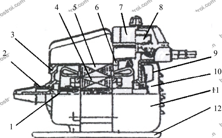
Рис. 2. Электропривод вибраторов ВИ-1-16, ВИ-1-17, ВИ1-13, ВИ-75
